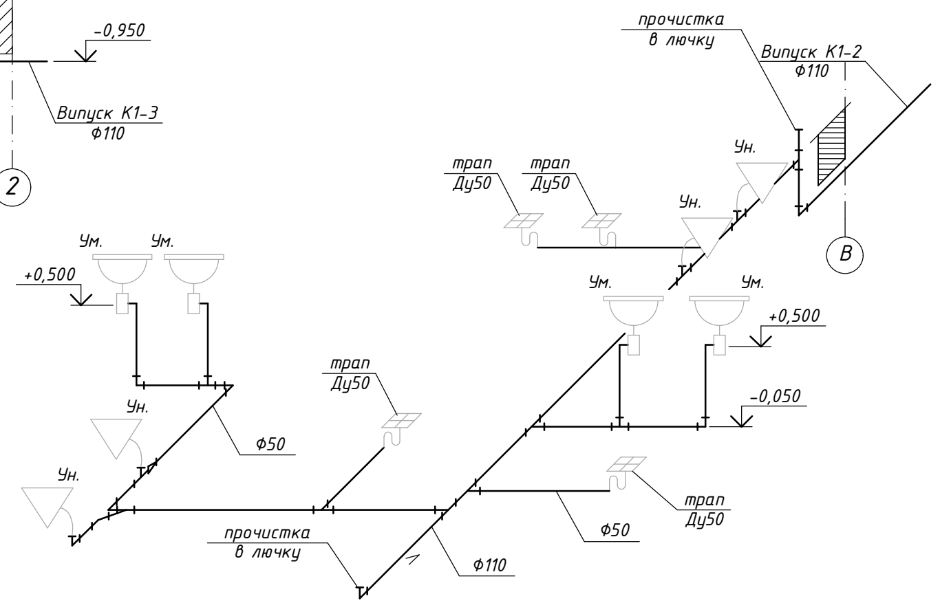
Схема К1-2
